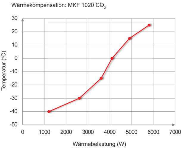
Wärmekompensationsdiagramm
