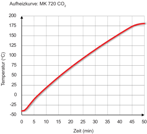
Aufheizkurve
