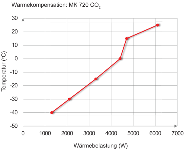
Wärmekompensationsdiagramm
