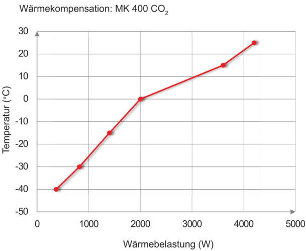
Wärmekompensationsdiagramm
