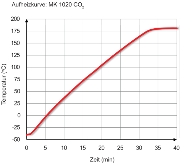
Aufheizkurve
